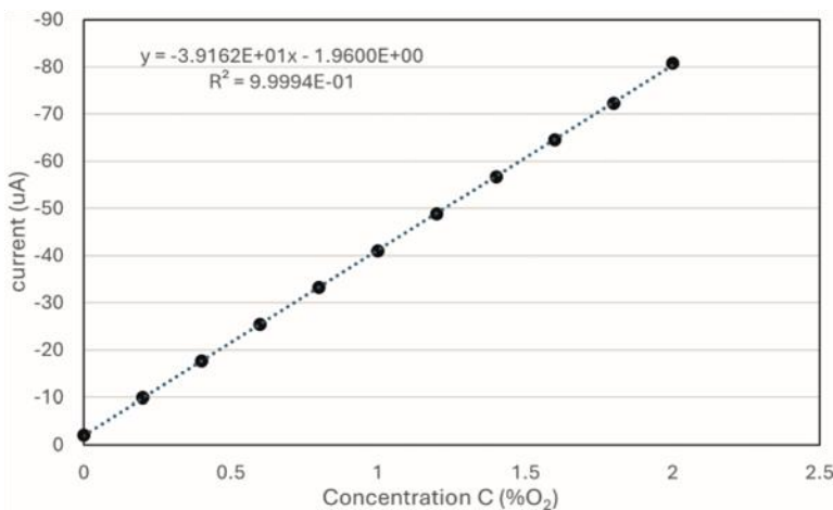
图 3. 0 ~ 2%O 2 的线性度
