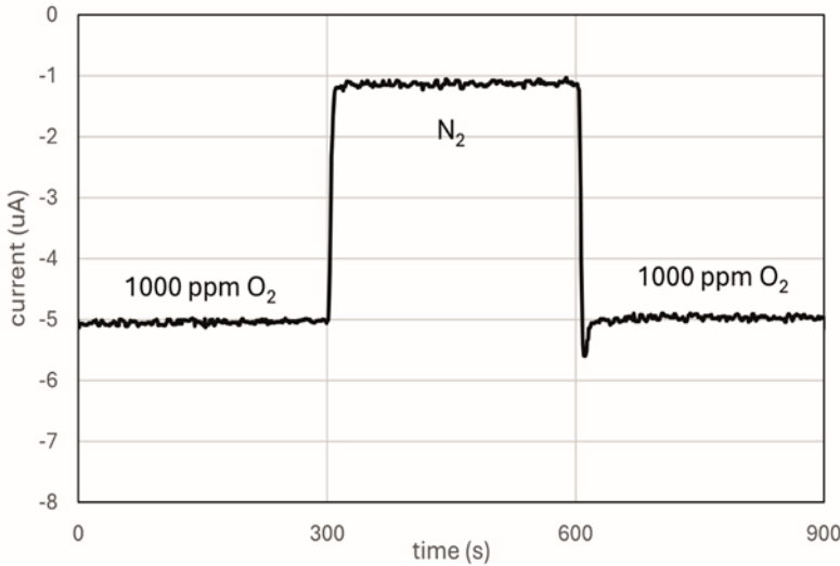
图 1.对 1000ppm O 2 的响应
