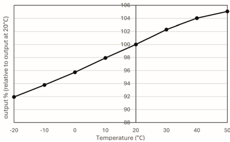
图 2.传感器的温度依赖性
